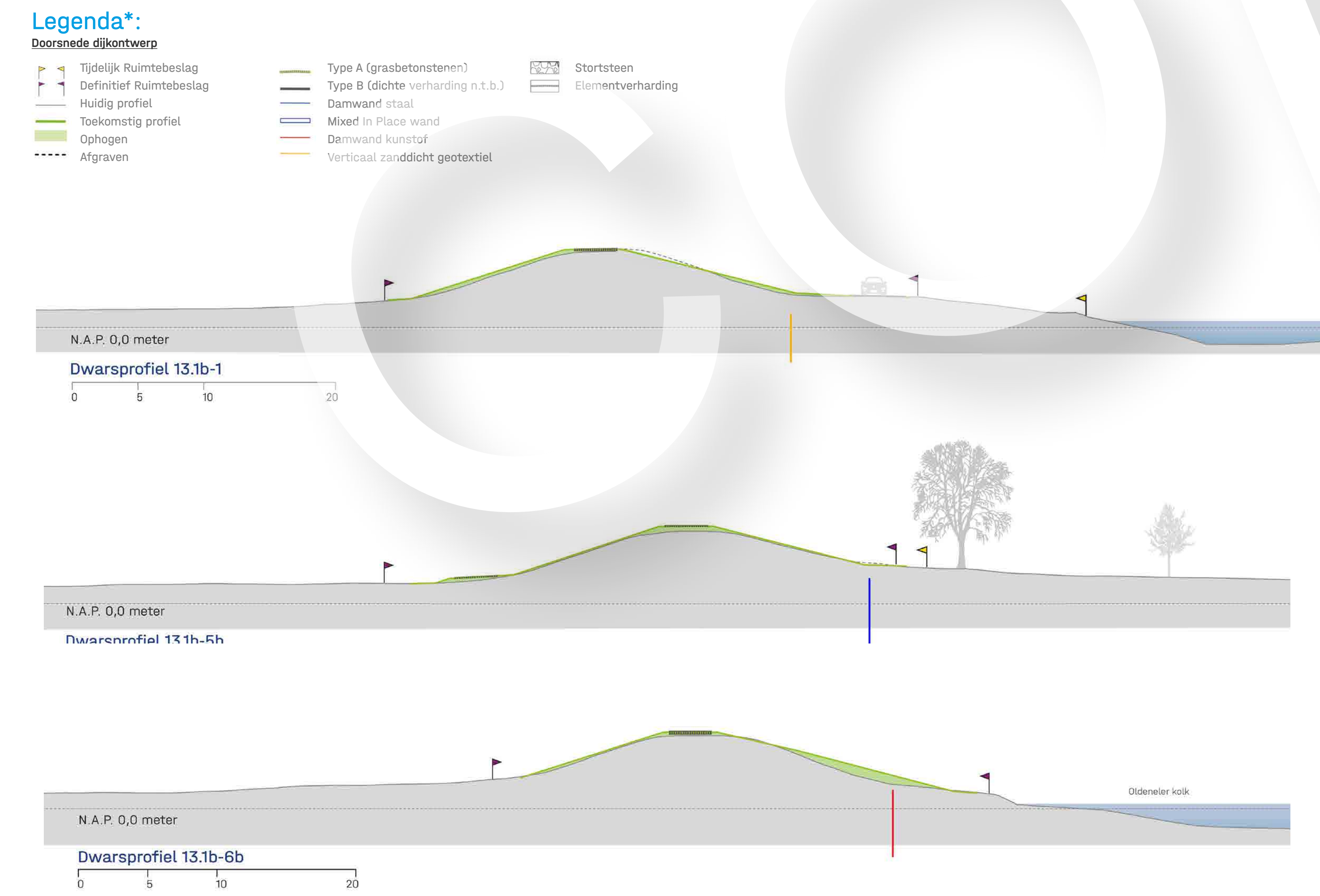
Doorsneden voorlopig ontwerp
