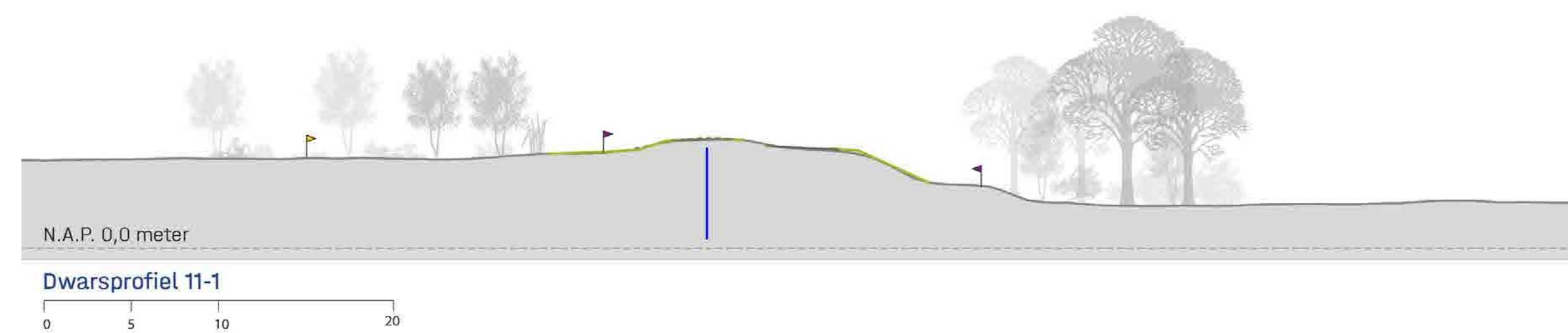
Doorsneden voorlopig ontwerp
